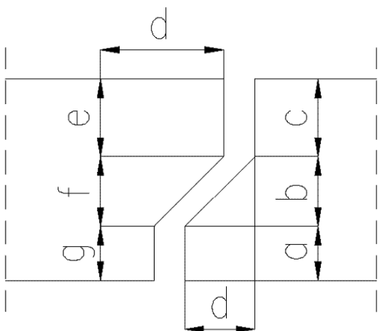
Rys.1. Typowe złącza między elementami prefabrykowanymi przepustów
