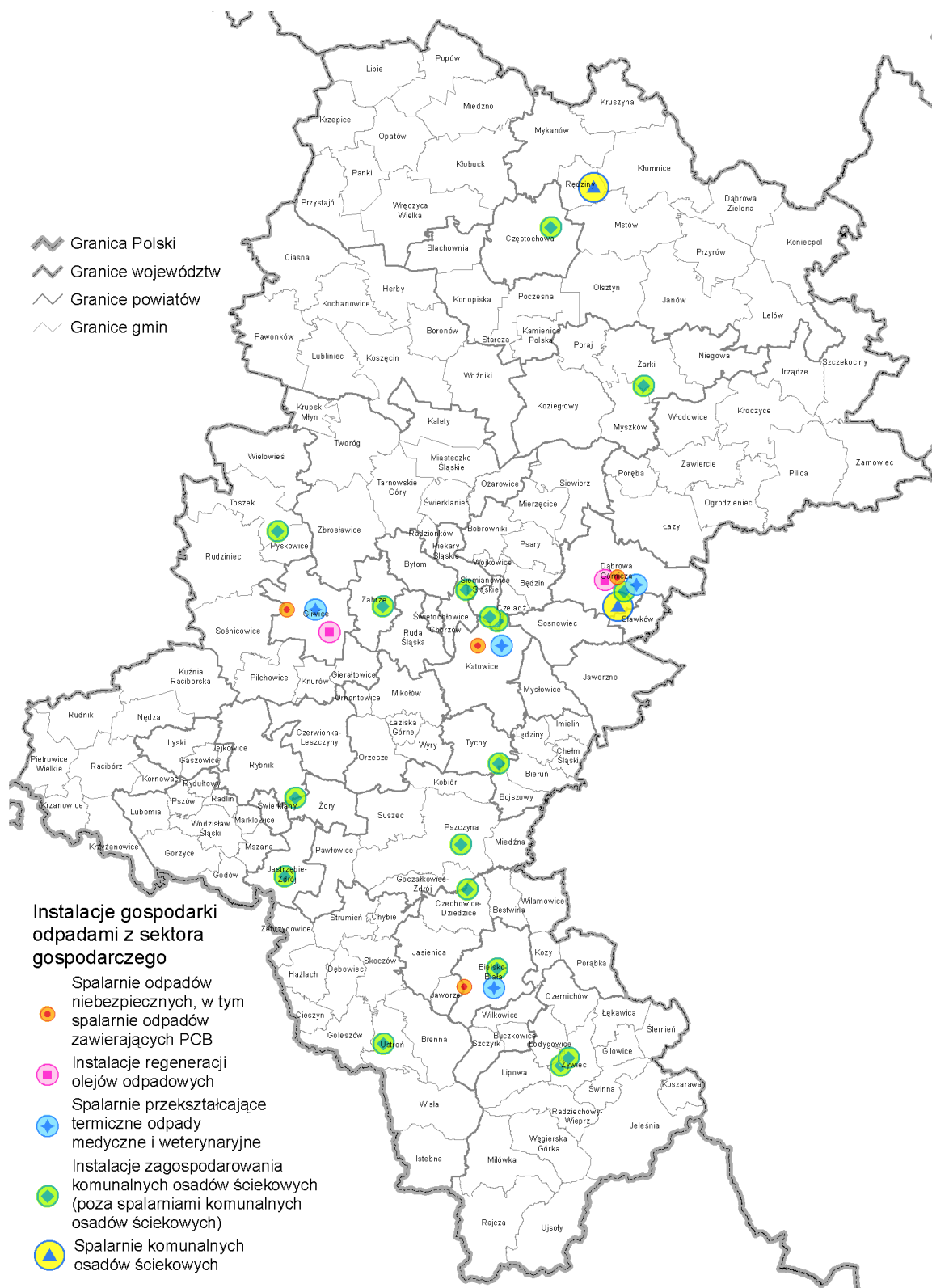
Rysunek 3-11 Spalarnie odpadów niebezpiecznych, odpadów medycznych i weterynaryjnych, komunalnych osadów ściekowych; instalacje regeneracji olejów odpadowych oraz instalacje zagospodarowania komunalnych osadów ściekowych
