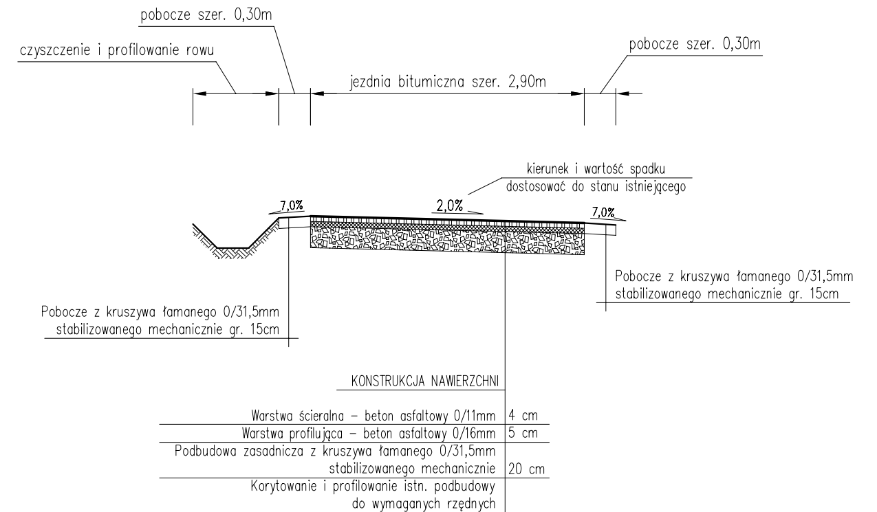
Przekrój typowy na odcinku od km 0+141,00 do km 0+250,00
